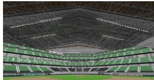
エスコンフィールド内 ホームベース側照明 (白い線は照明の光のイメージ)
