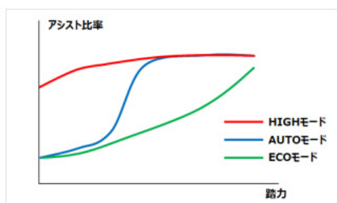
GXドライブユニット搭載XEALT M5のアシスト特性
